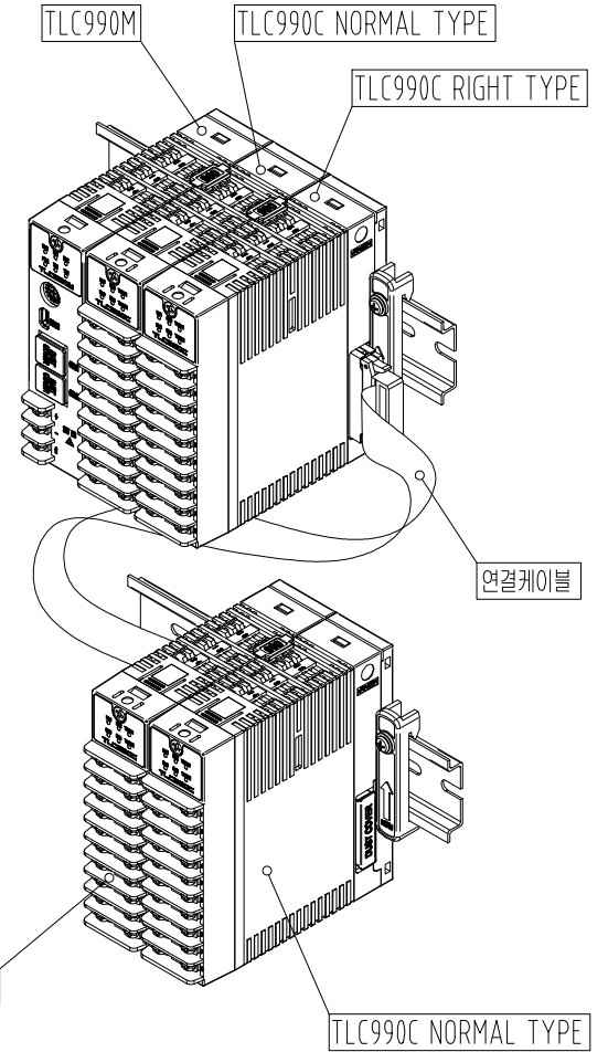
협소공간에서 케이블을 이용한 설치
