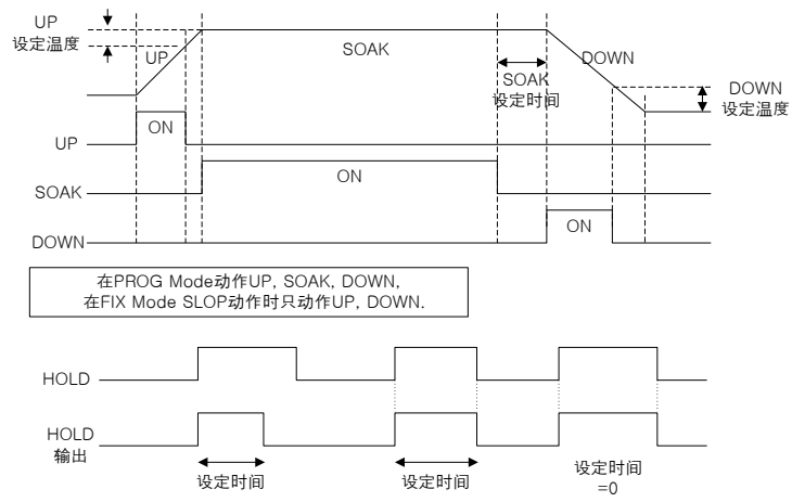
(图 23 : UP, SOAK, DOWN, HOLD 输出 例)
