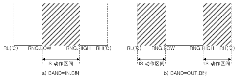
(图 21 : INNER SIGNAL 区间例)
