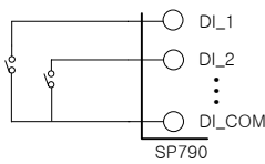
▲ RELAY 接点输入时
