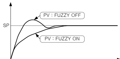
(图 10：根据FUZZY功能 控制OVER SHOOT)
