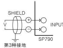
(2) 直流电压 输入(DC VOLTAGE INPUT)
