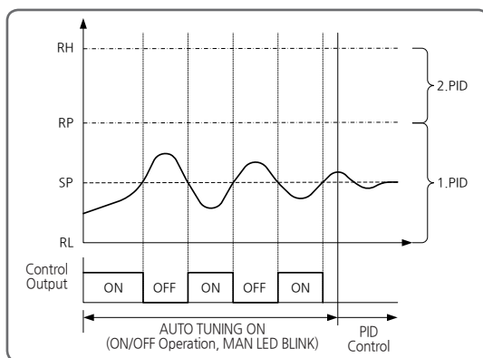
[Fig.2] Auto Tuning
