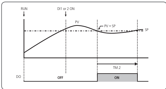
[Fig.39] TM.S : DI1 or 2
