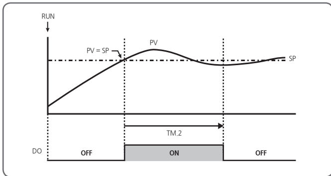
[Fig.38] TM.S : RUN
