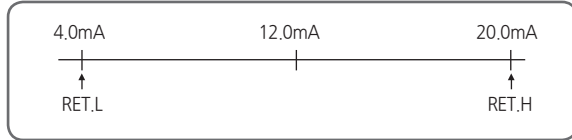
[그림10] 전송출력의 종류가 'PV' 또는 'SP'일 경우의 출력
