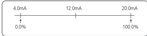
[그림11] 전송출력의 종류가 'MV'일 경우의 출력
