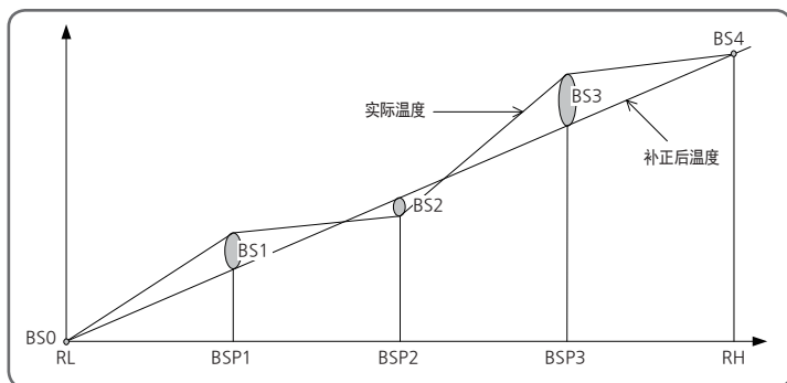
[图1] 区个别输入修正(BIAS)设定例
