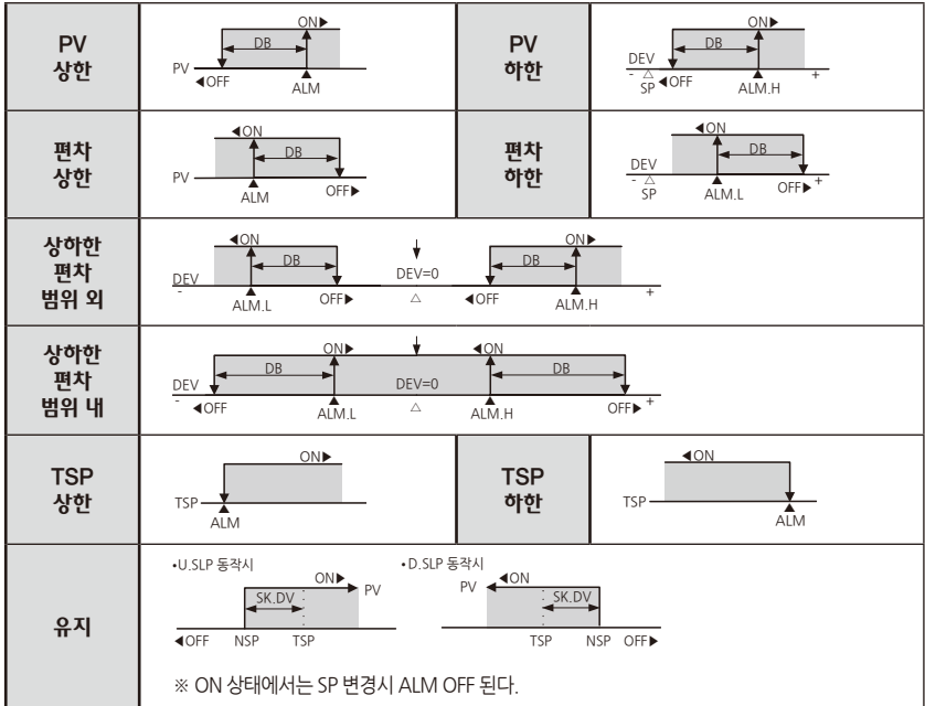
[그림20] 경보 동작
