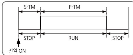
[그림14] 운전 예약 기능
