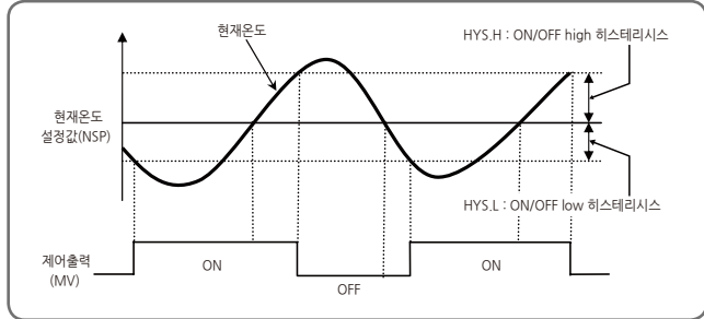
[그림19] ON/OFF 제어
