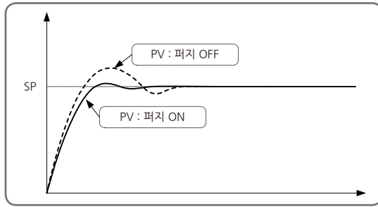
[그림6] 퍼지 기능에 의한 오버슈트(OVER SHOOT) 억제
