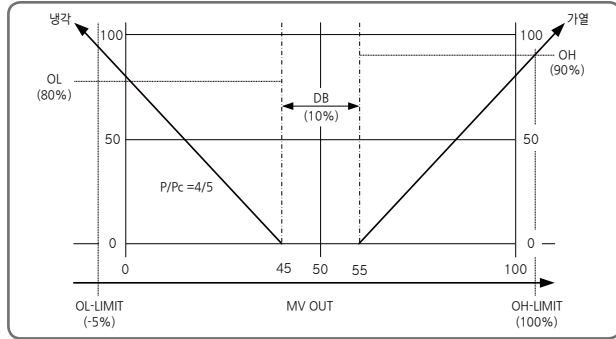
[그림9] 가열과 냉각이 모두 PID 제어인 경우 예
