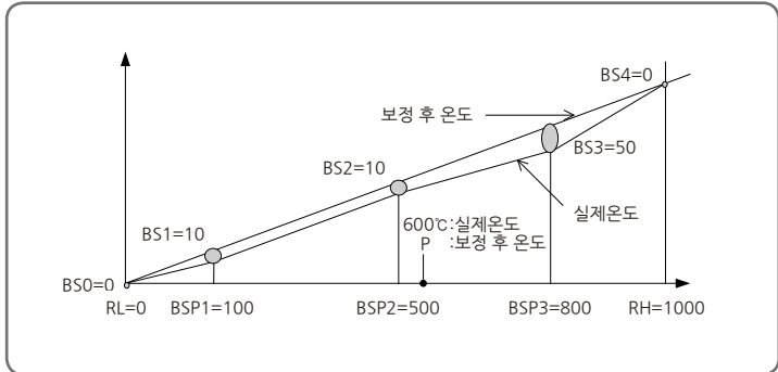
[그림16] 입력 보정 수식 예
