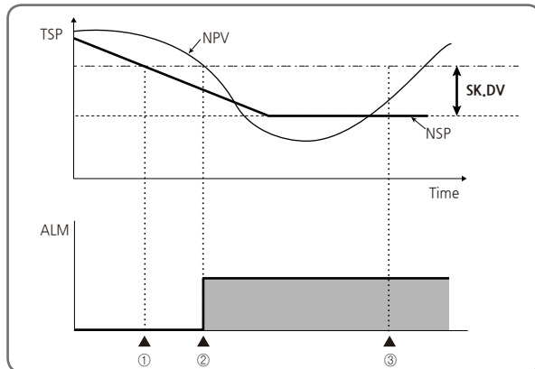
[그림22] DOWN SLOPE( \ : SP 하강변화중) 동작시
