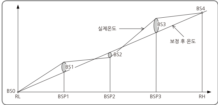
[그림15] 구간별 입력 보정(BIAS) 설정 예
