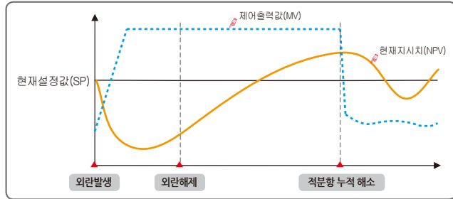
[그림4] 과적분방지 기능이 없는 경우
