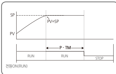
[그림12] PV=SP 모드 동작
