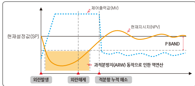
[그림5] 과적분방지 기능이 있는 경우
