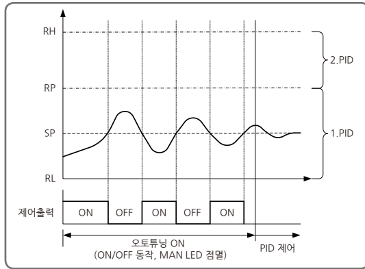
[그림1] 오토튜닝
