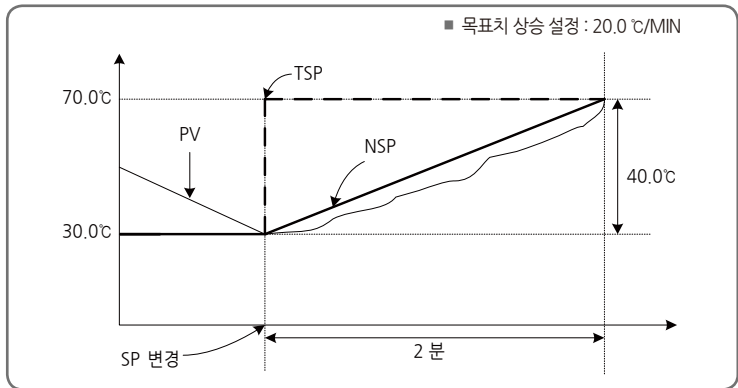
[그림3] 변화율(SLOPE) 동작
