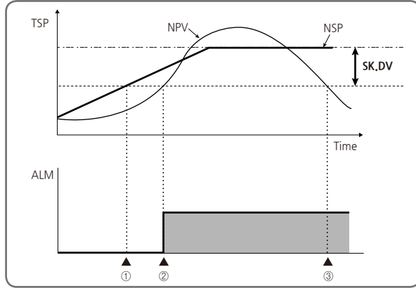
[그림21] UP SLOPE( / : SP 상승변화중) 동작시
