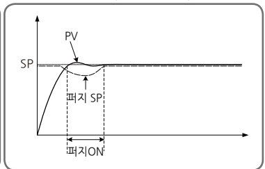
[그림8] 퍼지 ON
