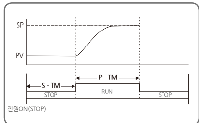
[그림13] S-TM 모드 동작
