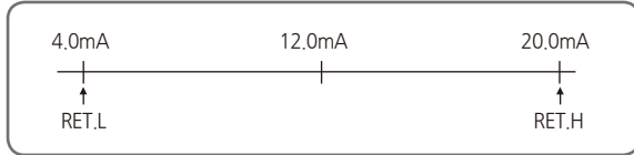
[그림23] 전송출력의 종류가 'PV' 또는 'SP'일 경우의 출력
