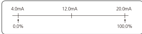
[그림24] 전송출력의 종류가 'MV'일 경우의 출력
