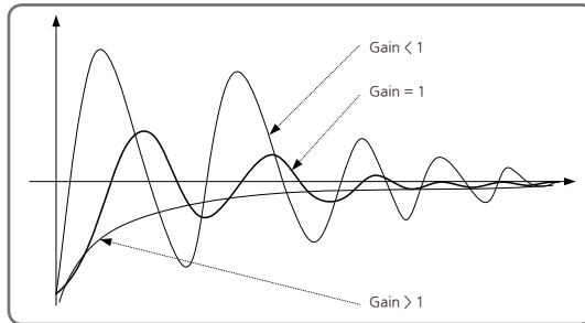
[그림2] 제어 시정수(AT GAIN)
