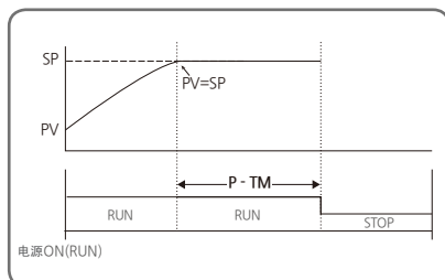
[图12] PV=SP模式动作
