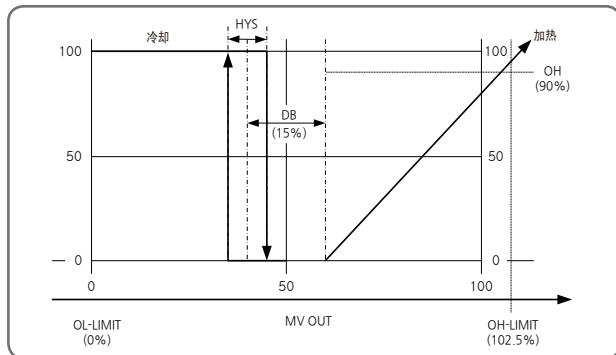
【图11】加热 = PID、冷却 = ON/OFF控制时的例子
