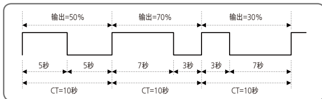
[图18] CT = 10秒时控制输出操作例
