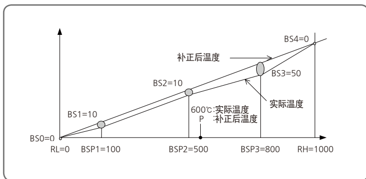
[图16] 输入修正式子例
