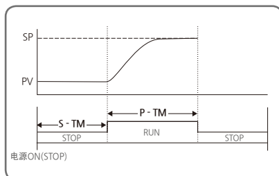
[图13] S-TM模式动作
