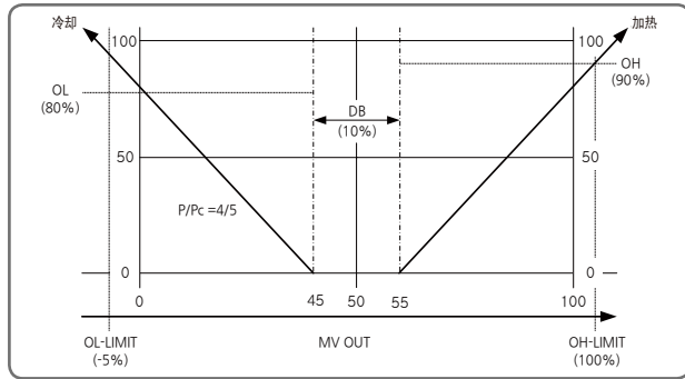
【图9】加热和冷却都是PID控制时的例子
