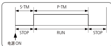
[图14] 运行预约功能
