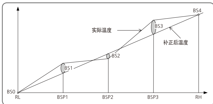
[图15] 区间接输入修正(BIAS)设定例
