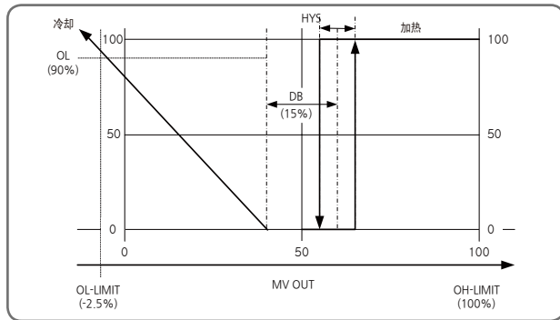
【图10】加热 = ON/OFF、冷却 = PID控制时的例子
