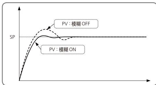
[图6] 由模糊功能抑制过冲
