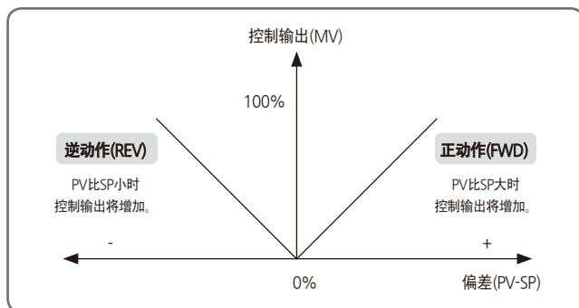
[图17] 正动作和逆动作
