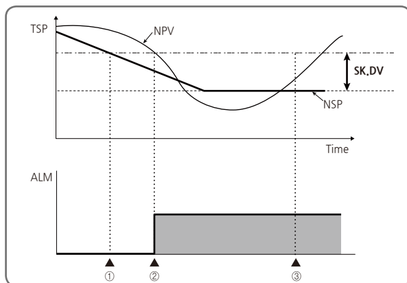
[图22] DOWN SLOPE(↘ : SP下降变化中)动作时
