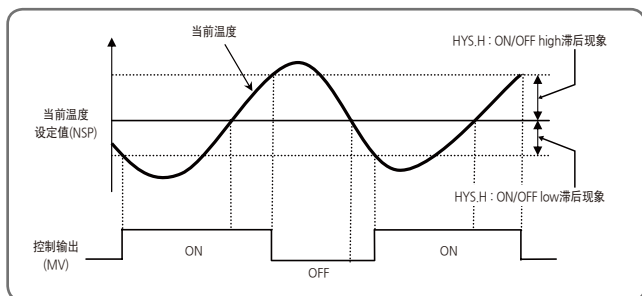
[图19] ON/OFF控制
